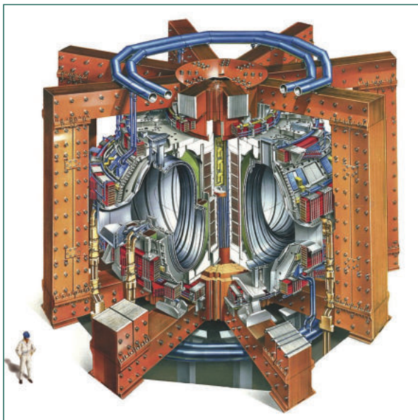
A fúziós reaktor szerkezeti rajza
